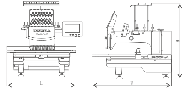
RCM-1501TC-7S L:744 W:856 H:820(mm)
